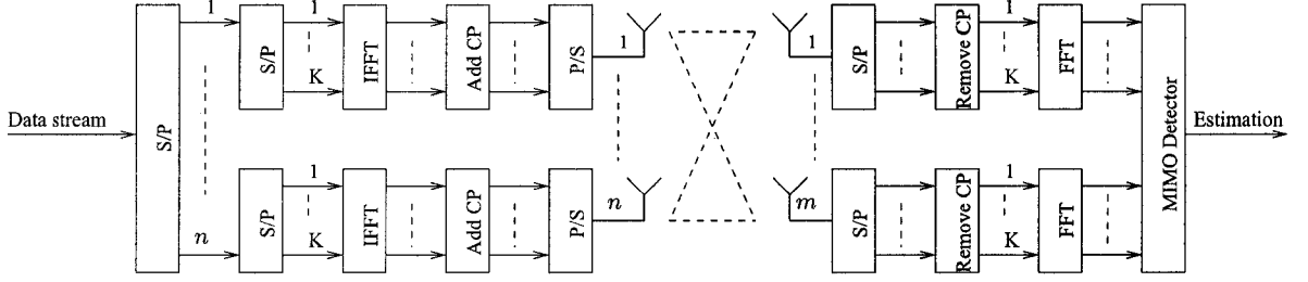
Fig. 2.11. System model.
