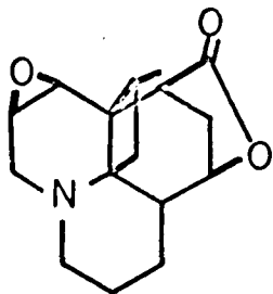
Annotinine
