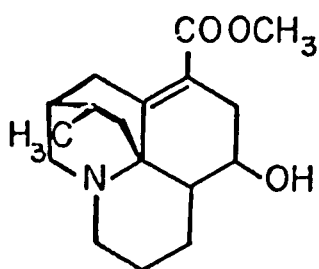
Annopodine 11
