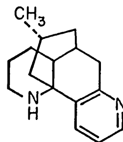
Lycodine 12
