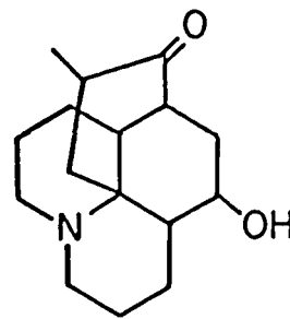
Annofoline 4
