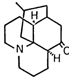
Lycopodine
