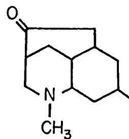
Luciduline 10
