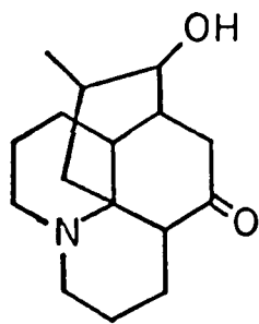
Clavolonine 3
