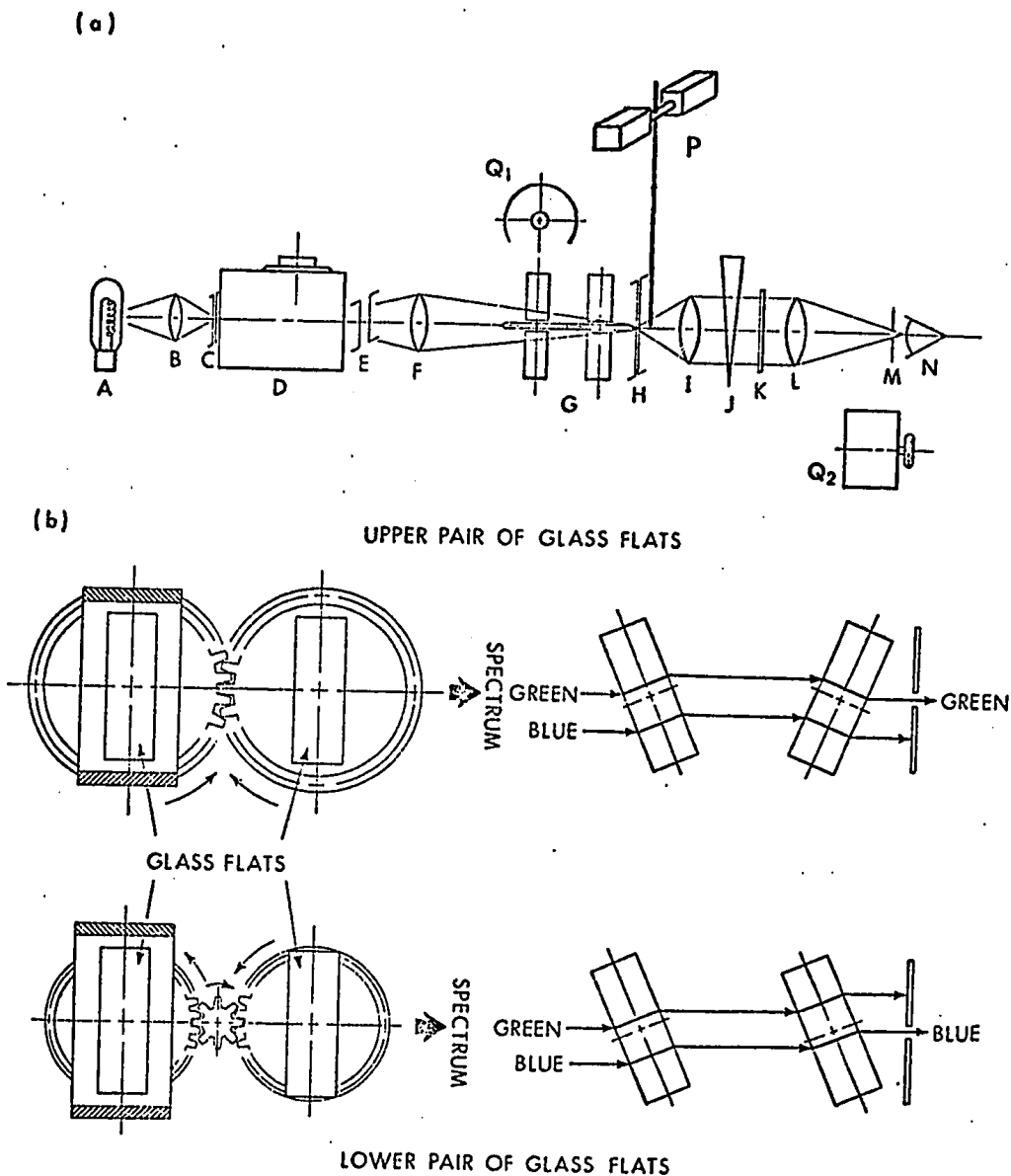
Fig. 1. Apparatus.
