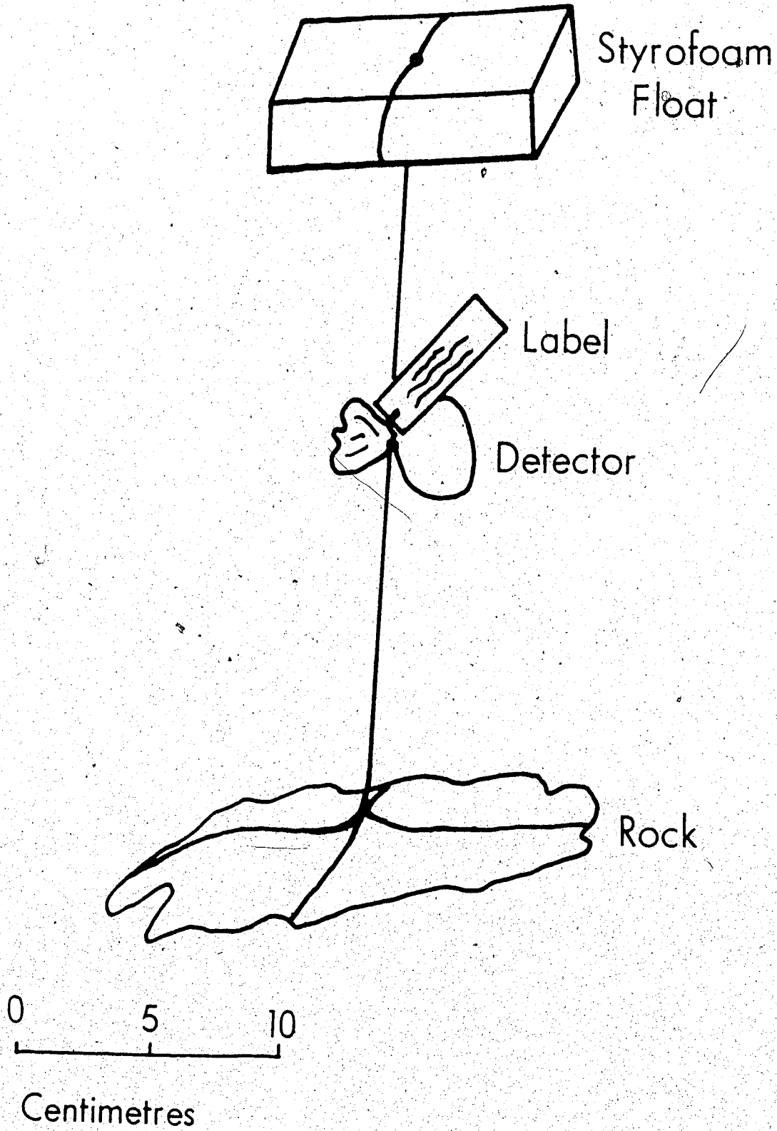
Figure 10 Lake bottom Detector
