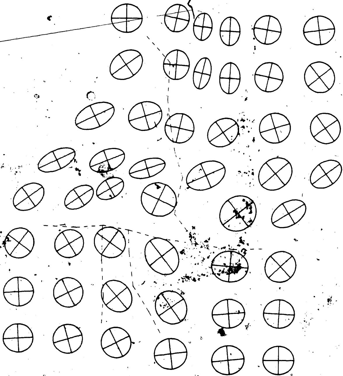
FIG. 9. Tissot's Elipses.
