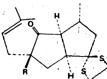
55 R = CHO
