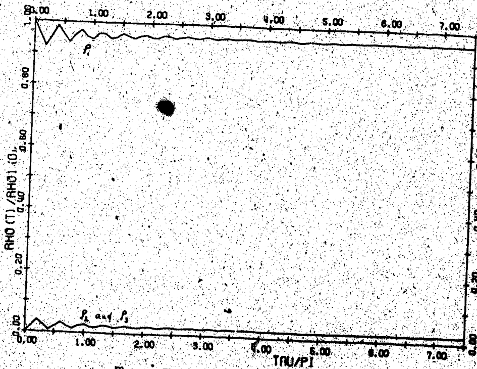
Fig. 2.8 (d) \frac{m_1}{m_2} = \frac{m_1}{m_3} = 0. ; r_2 = r_3 = \delta = U_1 = 1. ; U_2 = 10.
