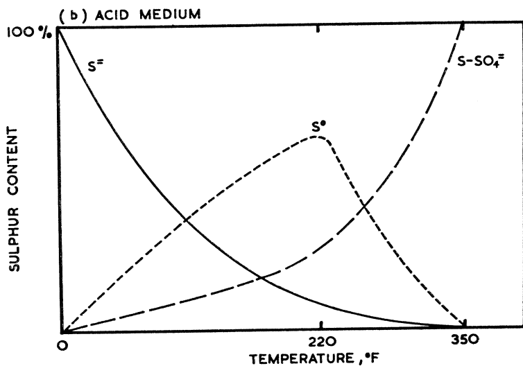
Рис. ч. 1. Оксидация сульфидной серки до сульфатів в амоніякальному і квасовому середовищі в залежності від температури.
