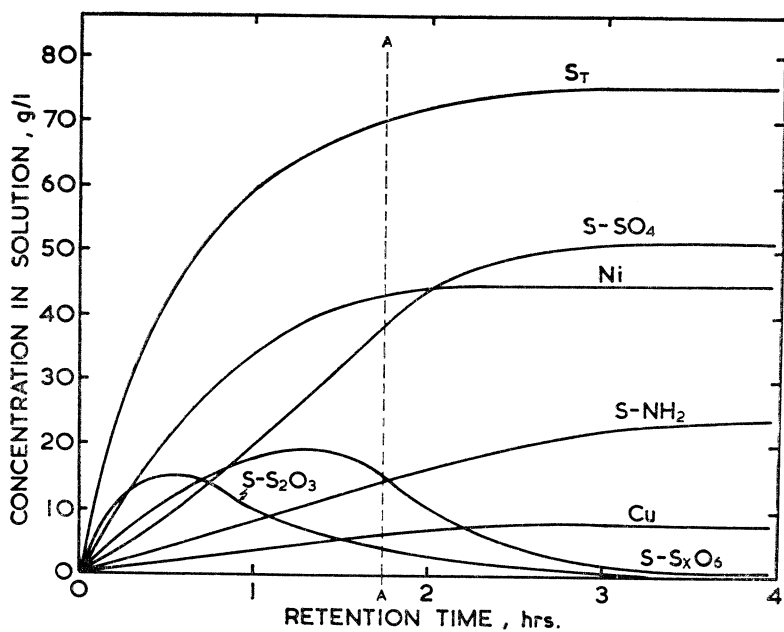
Рис. ч. 2. Швидкість вилуговлювання нікелевого концентрату в амоніякальному розчині.
