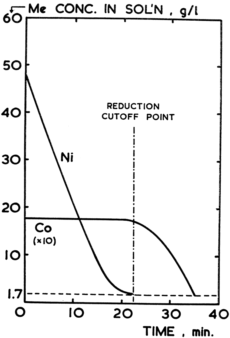
Рис. ч. 4. Швидкість редукції нікелю і кобальту з амоніякально-сульфатного розчину у великому продукційному автокляві. Умови редукції: 350 фунтів на квадратому стопу водню, 350 Ф.
