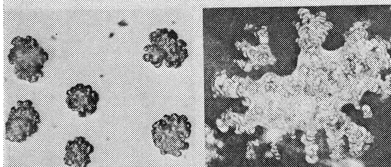
Прокатний порошок нікелю і його перекрій
