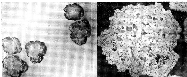
Стандартний порошок нікелю і його перекрій
