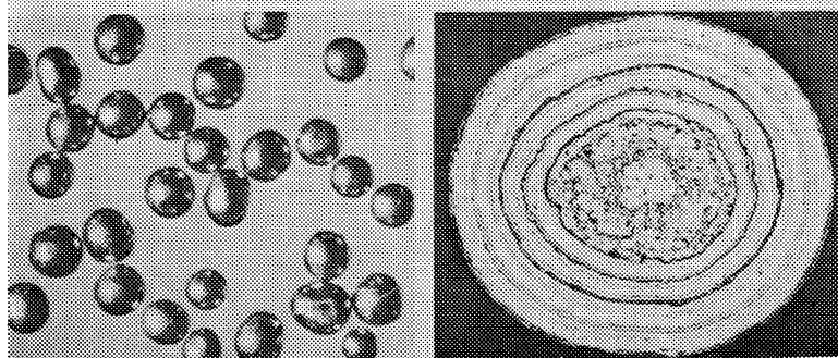
Сферичний порошок нікелю і його перекрій
