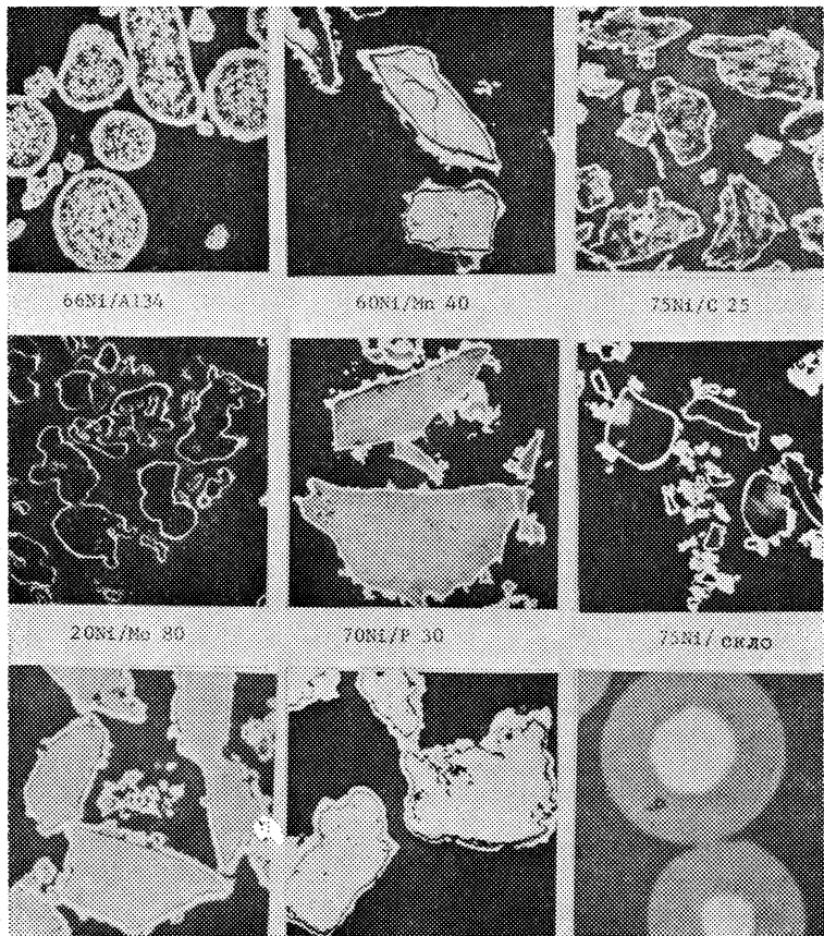
Рис. ч. 6. Покриті порошки приготовані методом редукції з водних розчинів. Різні матеріяли у порошковій формі покриті ніклем, кобальтом або оксидом молібдену. Порошки в перекрою.
