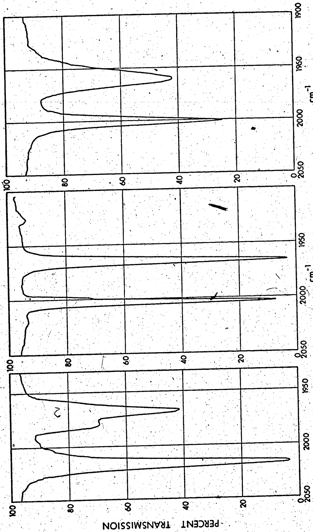
(Et_2Ge)_2Fe_3(CO)_9 Figure 9
