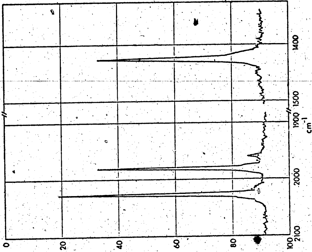
trans -CpRe(CO) 2 (GeCl 3 )D
