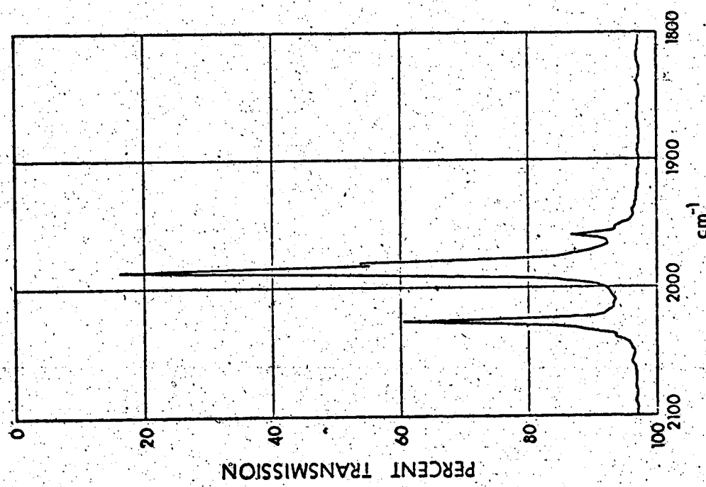
trans -CpRe(CO) 2 (GeCl 3 )H
