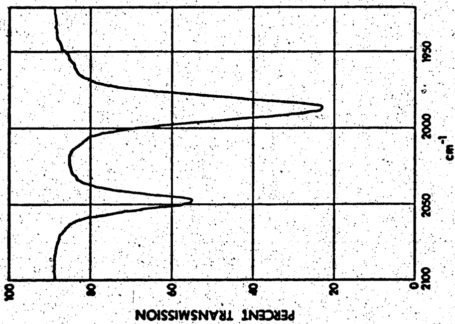
trans -CpRe(CO) 2 I 2
