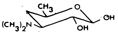
D-Desosamine
