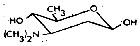
D-Angolosamine
