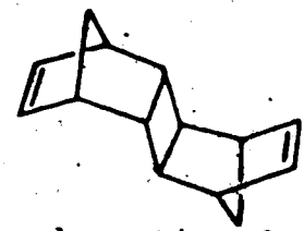
endo-anti-endo
