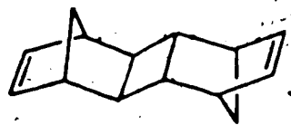
exo-anti-exo
