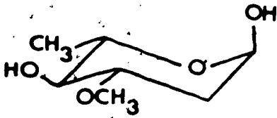
L-Oleandrose
