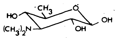
D-Mycaminose
