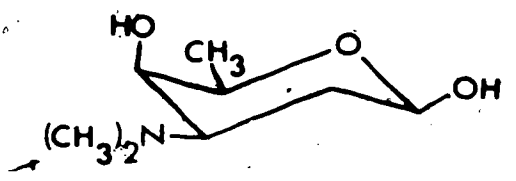
D-Rhodamine
