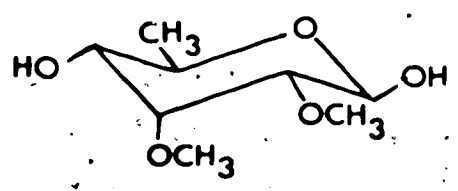
D-Mycinose
