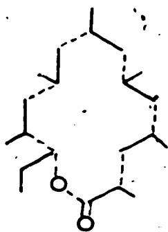
erythromycin
