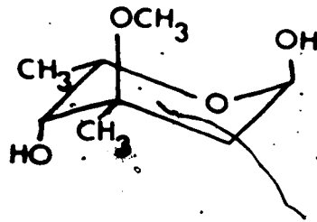
L-Arcanose
