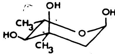
L-Mycarose
