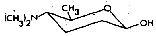
D-Forosamine
