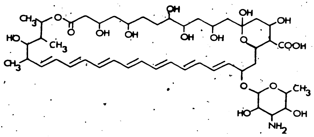
Amphotericin B
