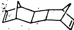
exo-anti-endo
