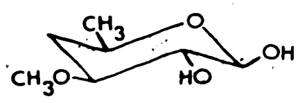
D-Chalcose
